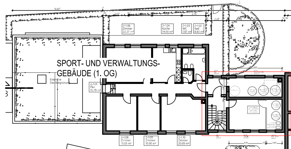
AUSSCHNITT GRUNDRISS 1. OG M. 1:50
