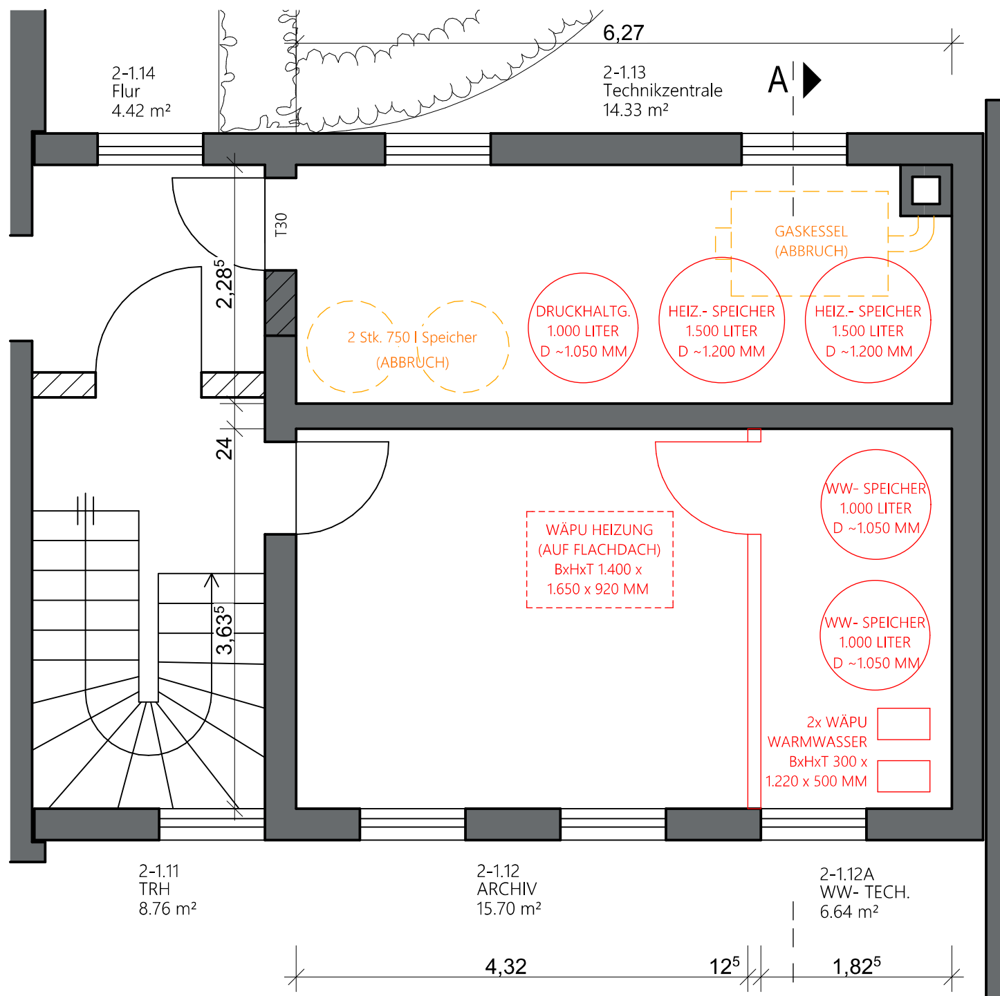
AUSSCHNITT GRUNDRISS 1. OG M. 1:50
